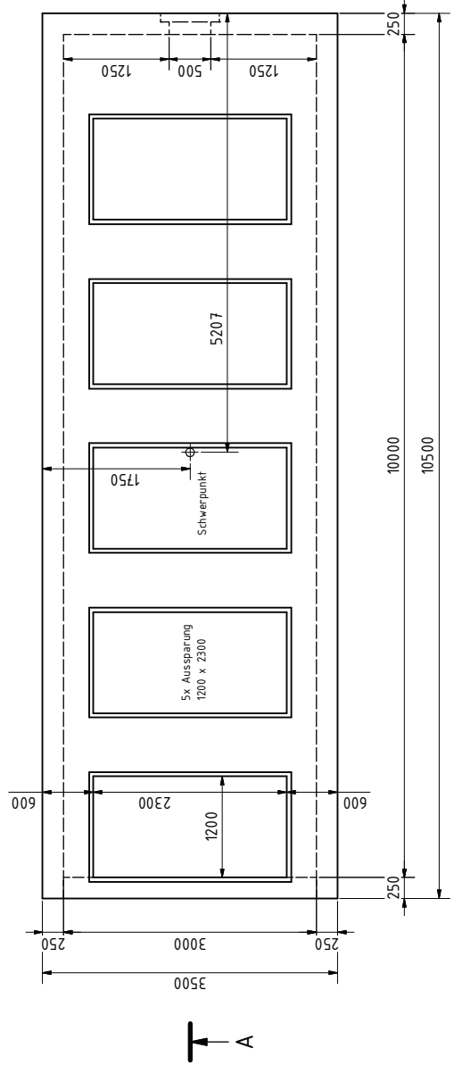
Grundriss ( 1 : 40 )
